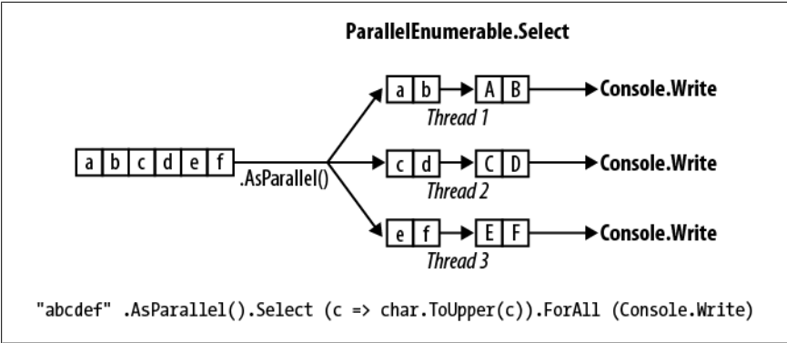
Figure 23-3. PLINQ ForAll
